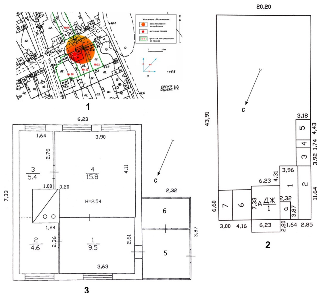
Ил. 1. Архив автора. Микрорайон Сумкино, ул. Дачная, 32. План усадьбы (1 — фрагмент плана мкр. Сумкино с участком возгорания; 2 — план участка с постройками (1А — дом с полисадником, 1 — крытый двор (а — крыльцо с тамбуром), 2 — первый гараж, 3 — хлев, 4 — коридор для подхода к сеновалу и входа в баню, 5 — баня, 6 — второй гараж, 7 — навес); 3 — план дома (1 — гостиная, 2 — кухня, 3 — спальня, 4 — зал, 5 — тамбур с летней кухней, 6 — чулан)).
